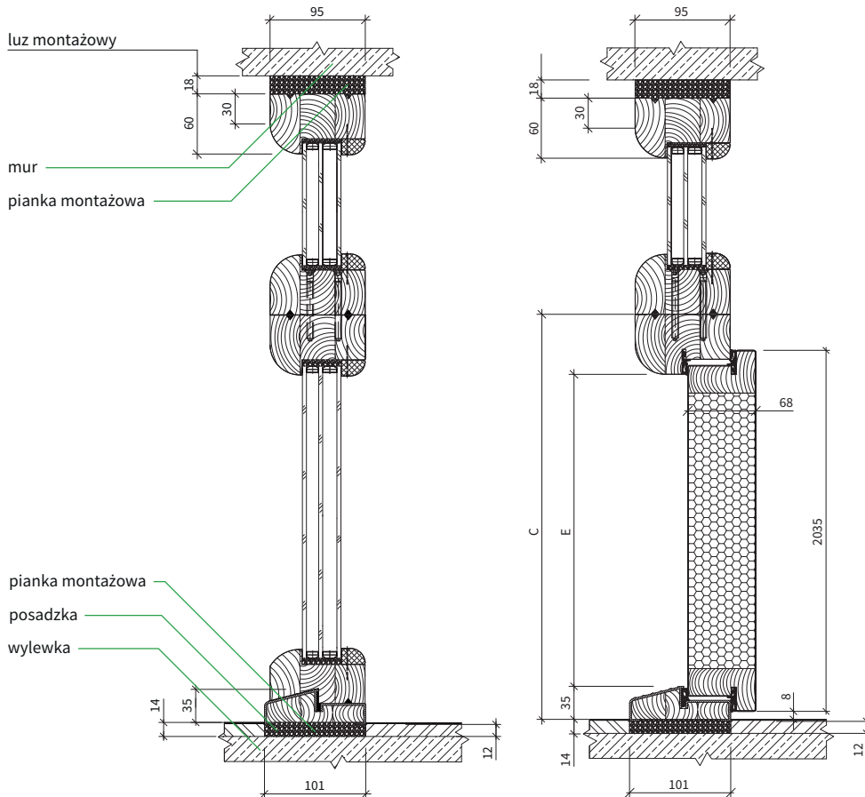
Przekrój przez dostawkę boczną
